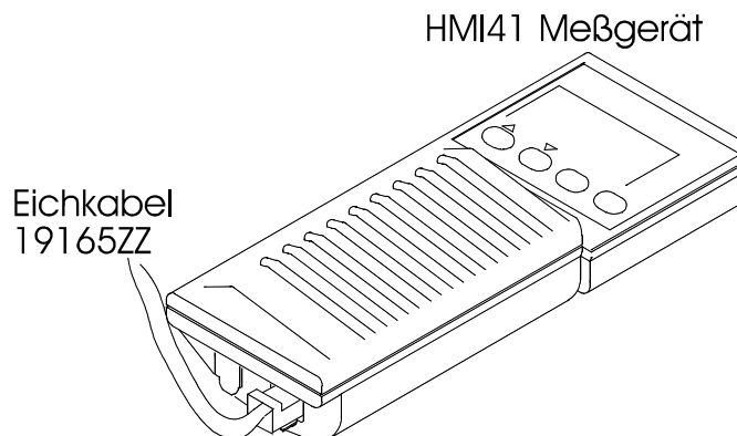
Abbildung 2.1 Position des Kalibriersteckers beim HMI41
