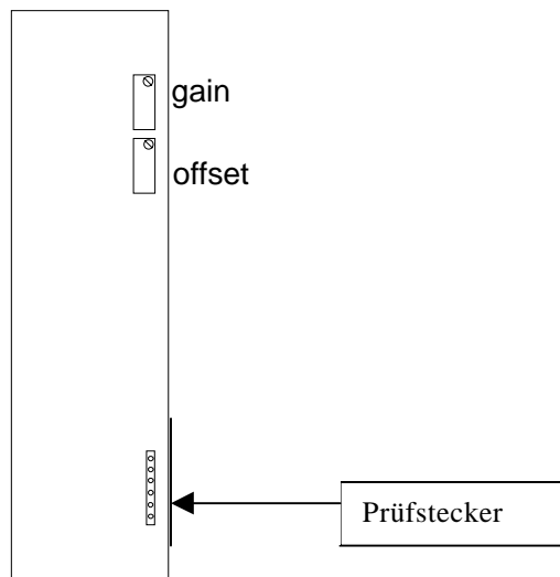
Abbildung 2.4 Kalibrierstecker und Potentiometer der HMD 20/30UB/YB - Meßwertgeber
